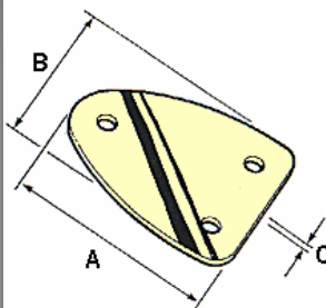
3xØ 4.5 mm holes
