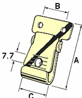
3xØ 4.5 mm holes
